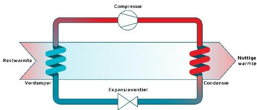
Compressiewarmtepomp, werkingsprincipe
